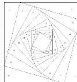
Рис. 8. Способ укладывания полос - «диафрагма». Базовый элемент – квадрат
